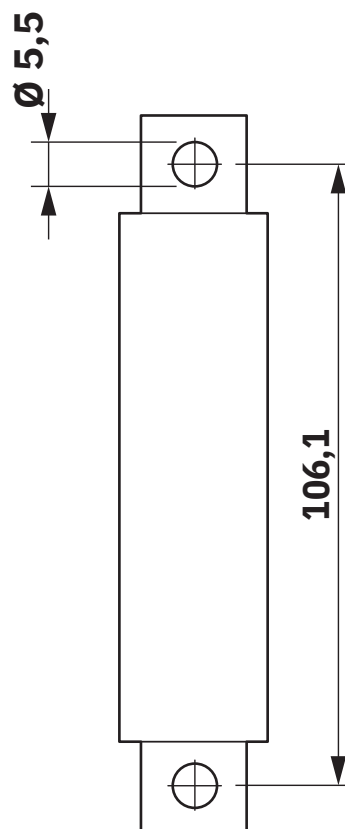
Disegno quotato
