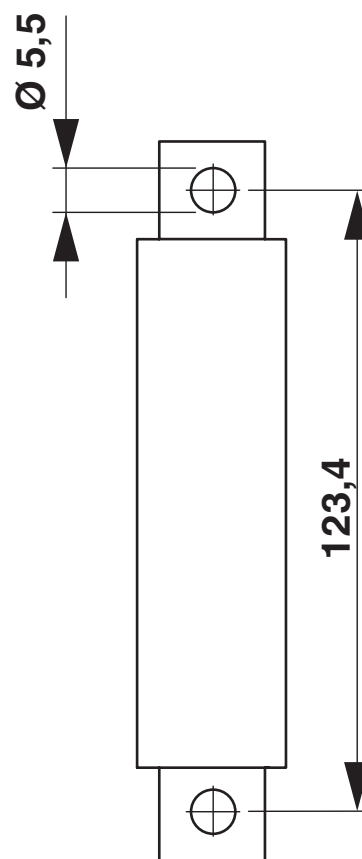
Disegno quotato
