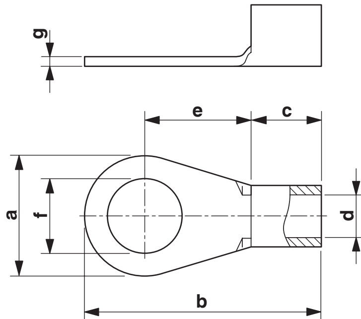
Disegno quotato
