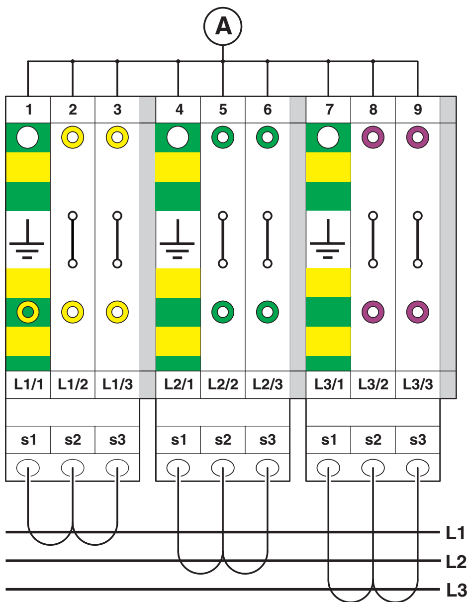
Disegno collegamento
