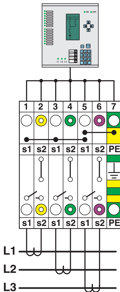
Disegno schema
