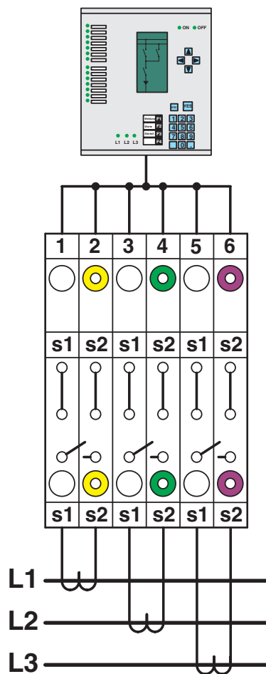
Disegno schema
