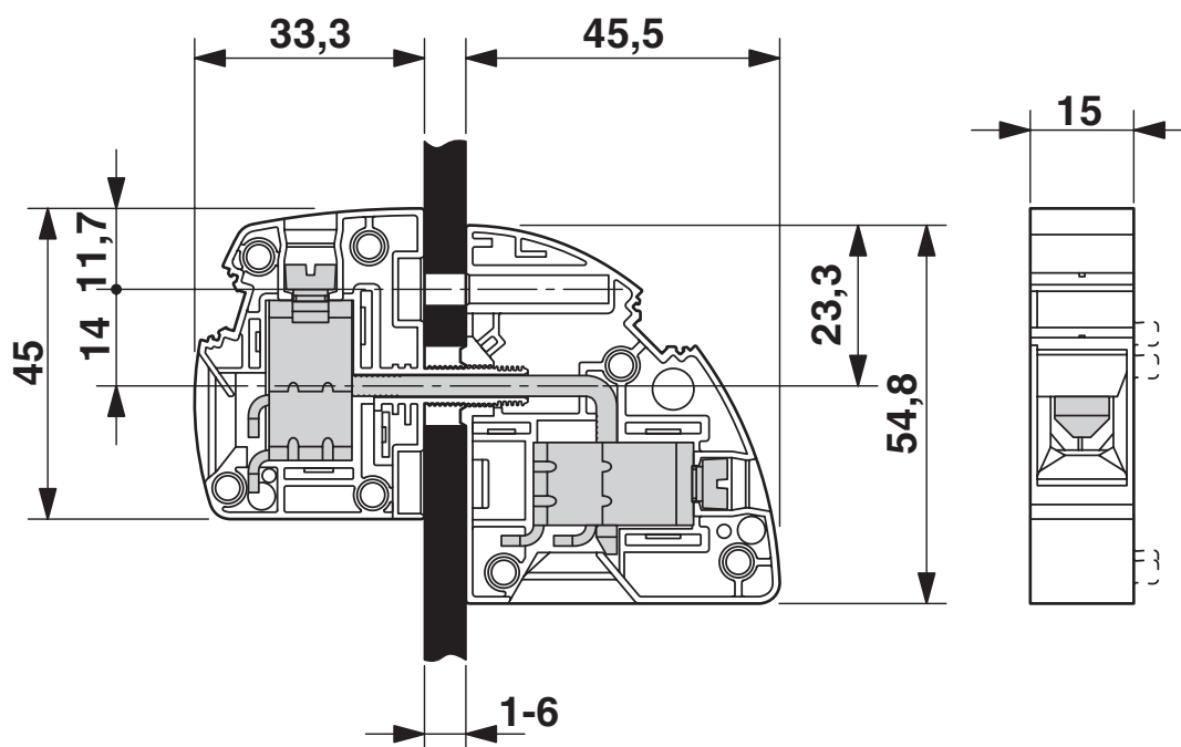
Disegno quotato
