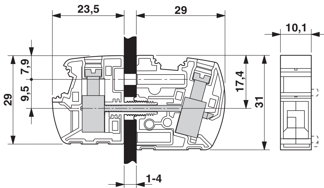
Disegno quotato
