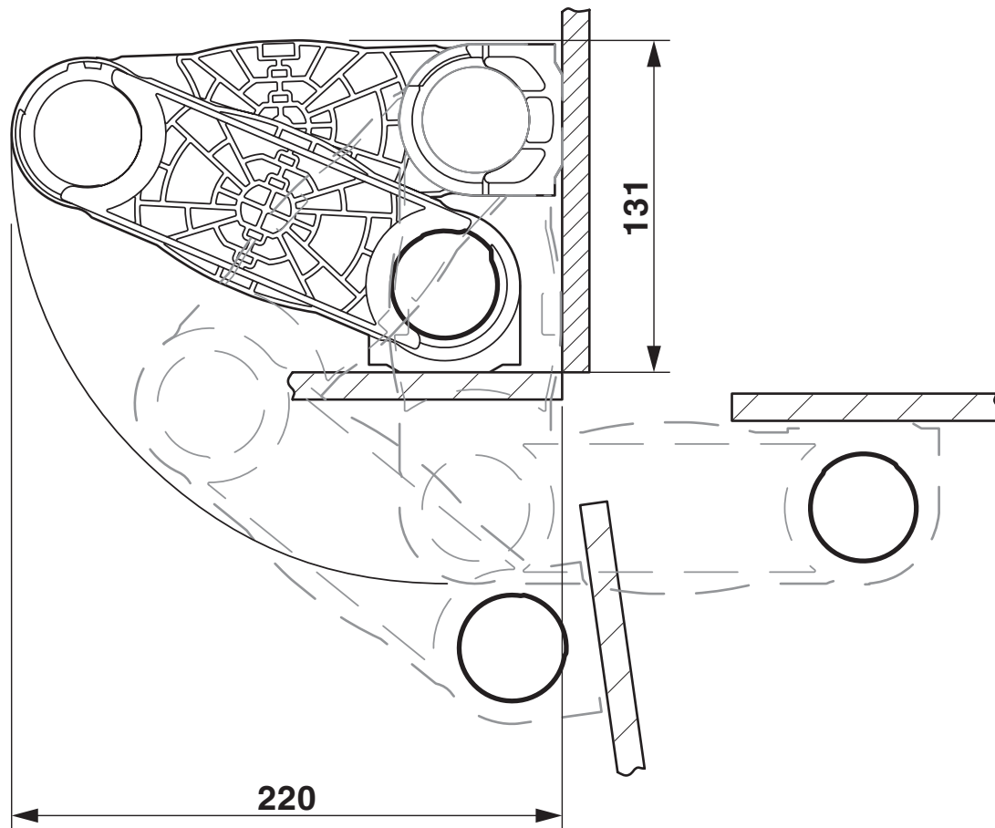
Disegno quotato
