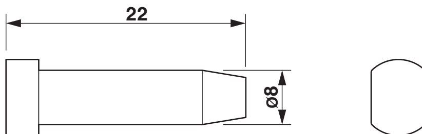
Disegno quotato
