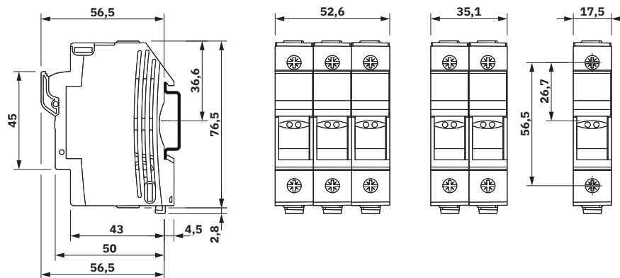
Disegno quotato
