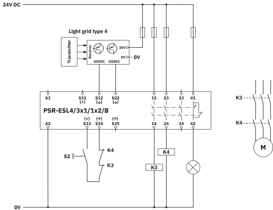
Schema di collegamento
