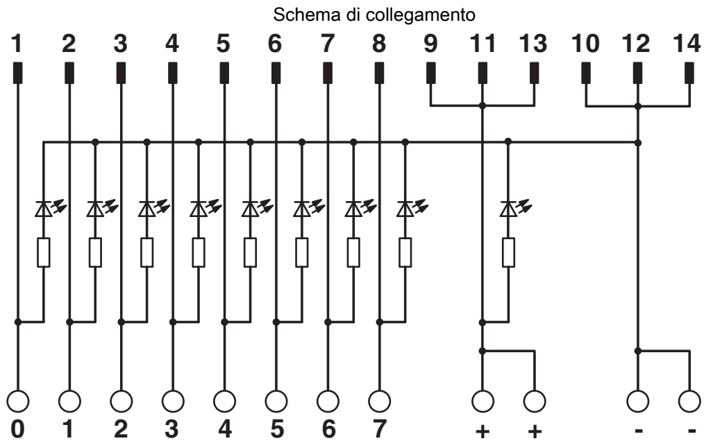
Schema di collegamento UM 45-FLK14/LA/PLC
