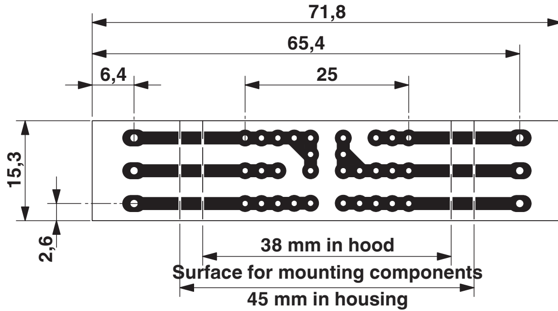
Disegno quotato
