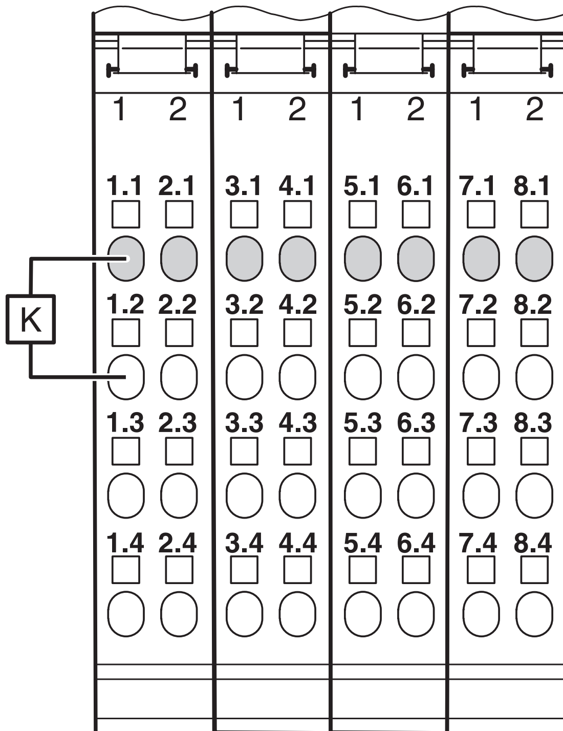
Disegno collegamento
