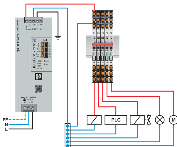
Disegno applicazione
