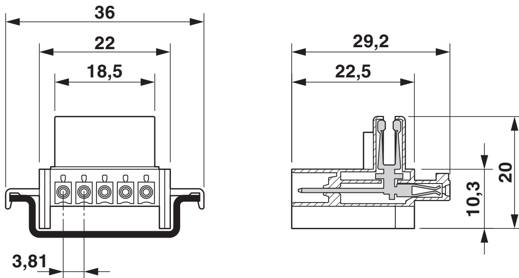
Disegno quotato
