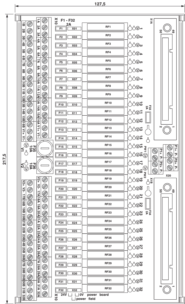
Disegno quotato
