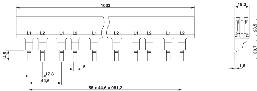
Disegno quotato
