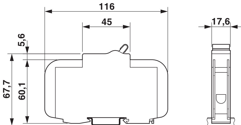
Disegno quotato
