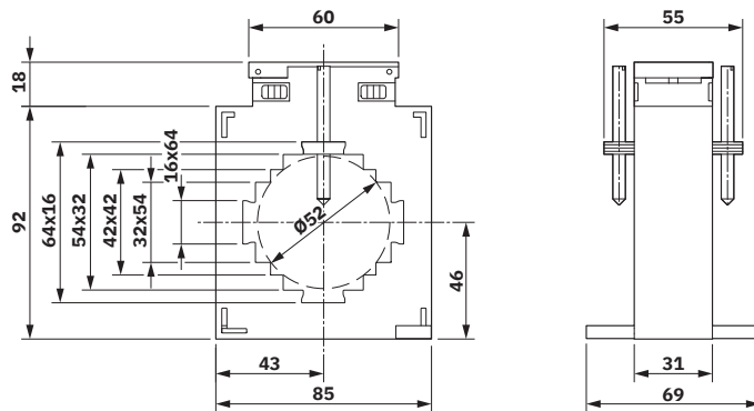
Disegno quotato
