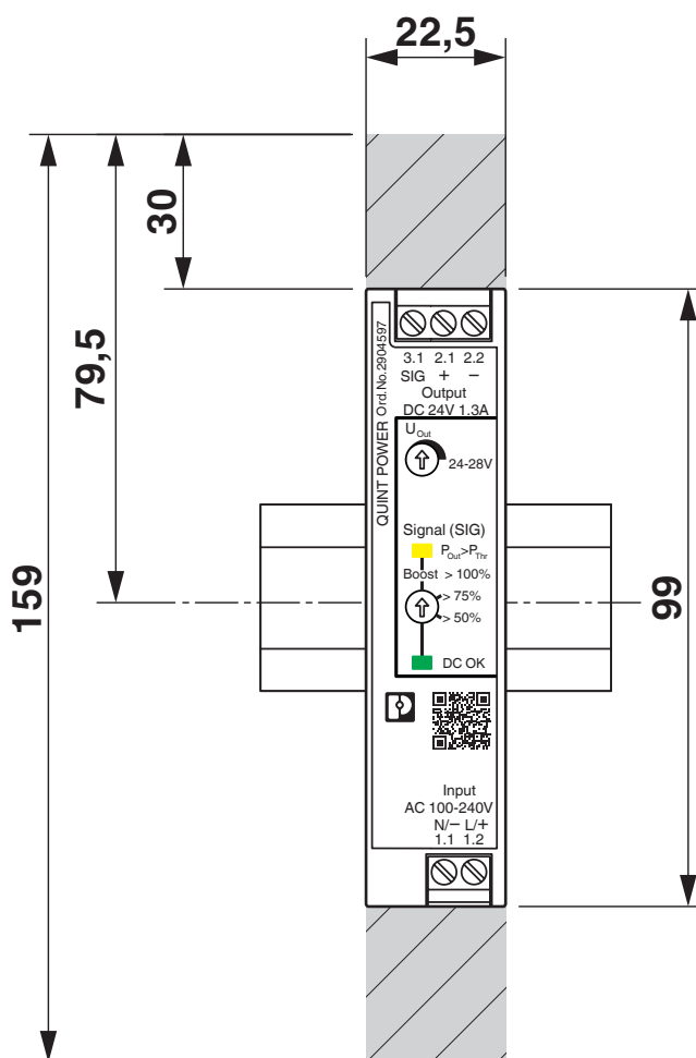
Disegno quotato
