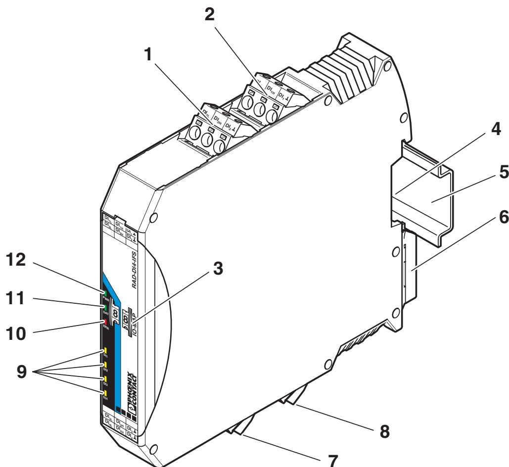
Disegno schema
