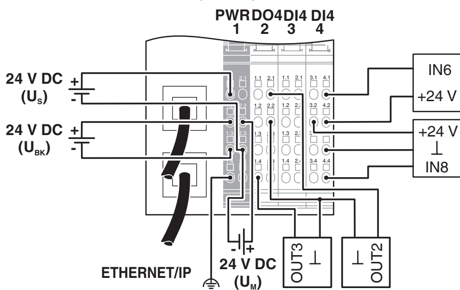
Disegno collegamento
