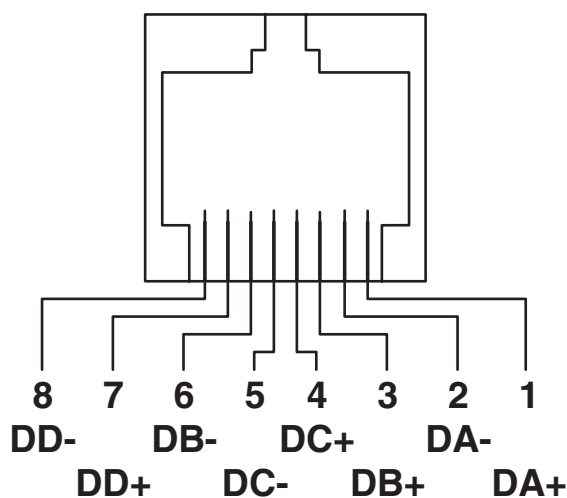
Disegno schema
