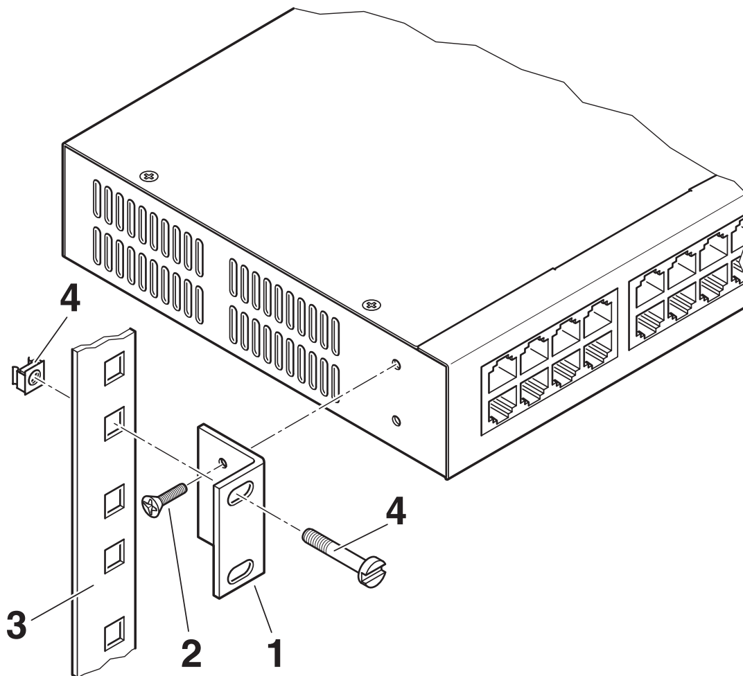
Disegno applicazione
