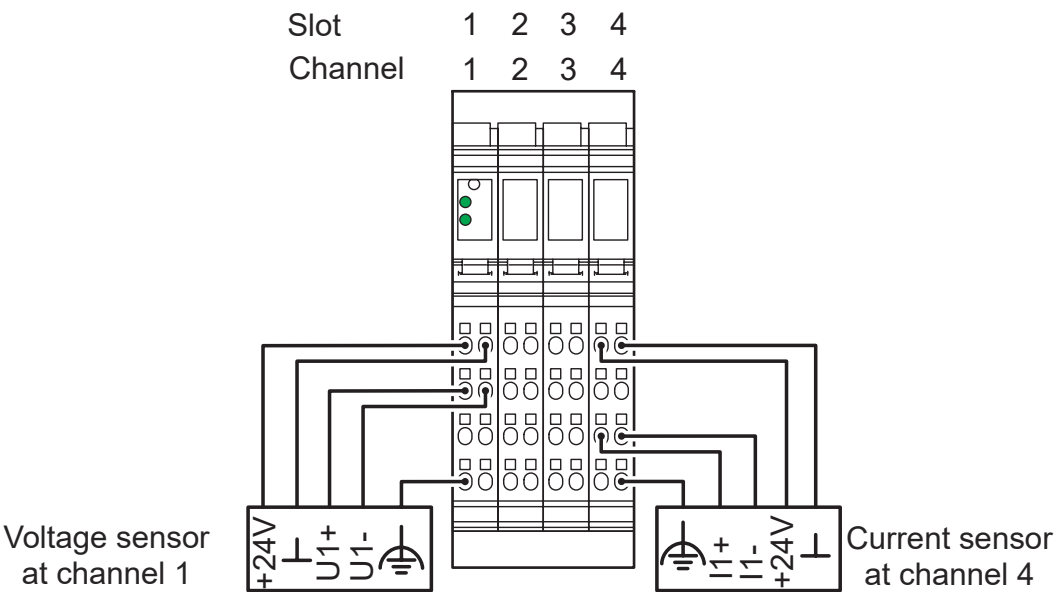
Disegno collegamento
