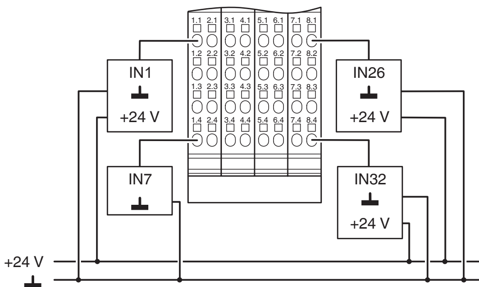
Disegno collegamento
