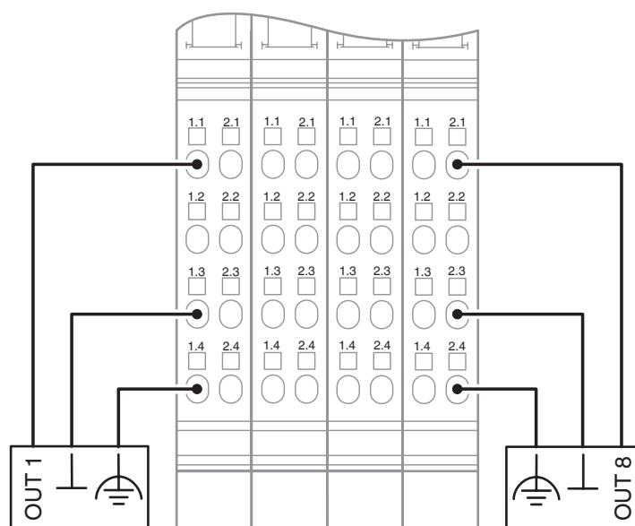
Disegno collegamento
