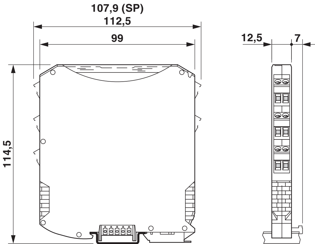
Disegno quotato
