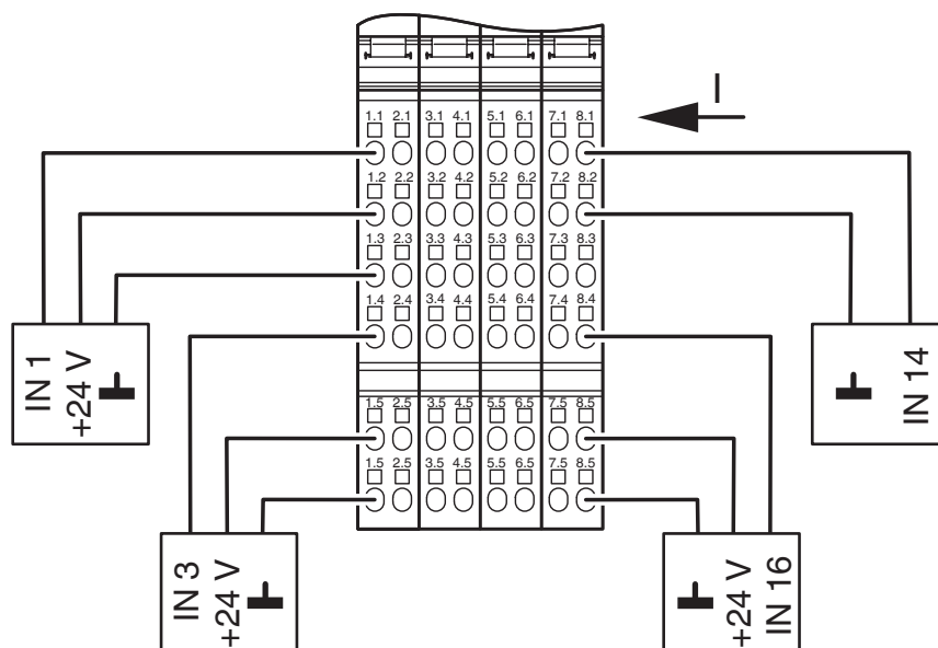
Disegno collegamento
