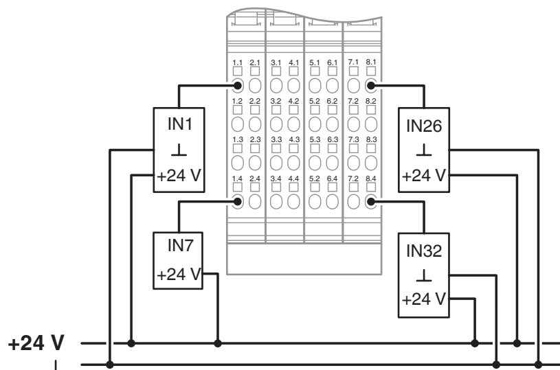
Disegno collegamento
