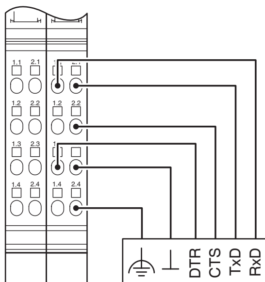
Disegno collegamento
