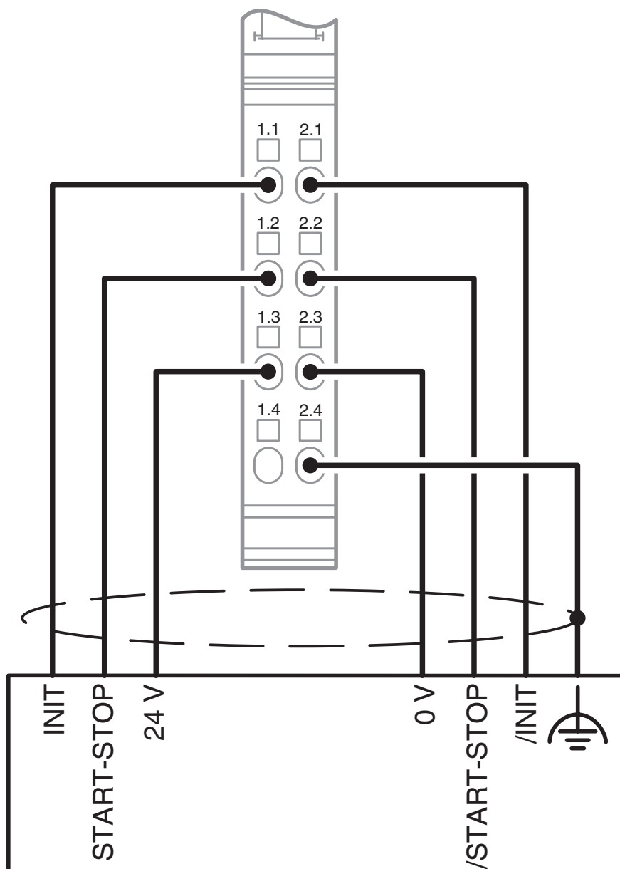
Disegno collegamento
