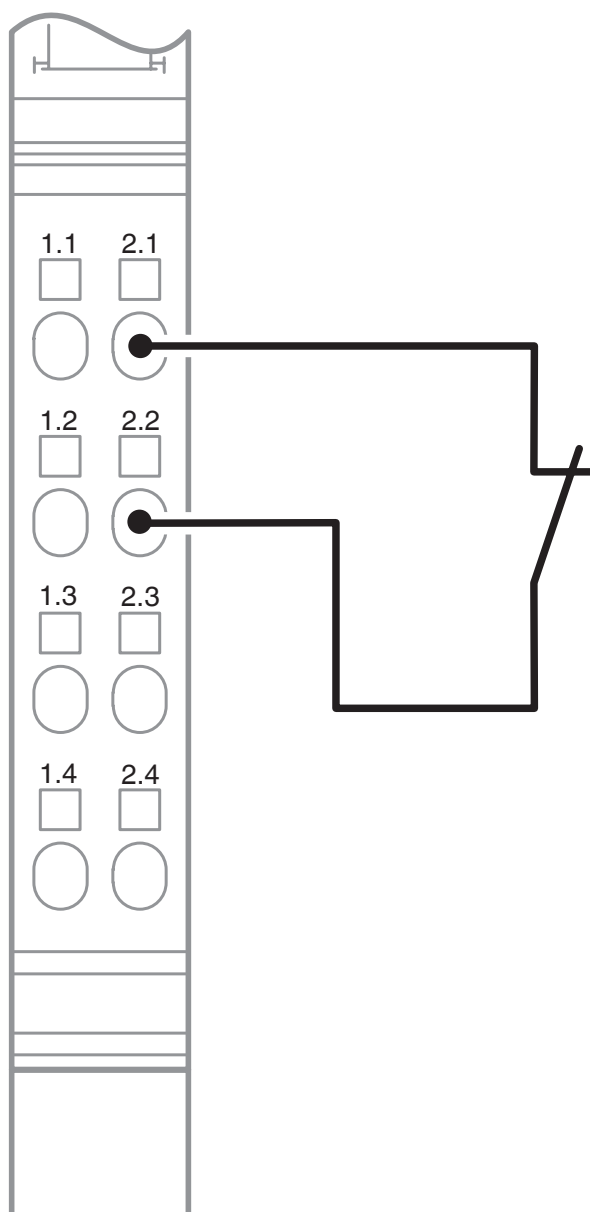
Disegno collegamento
