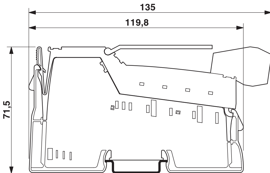
Disegno quotato
