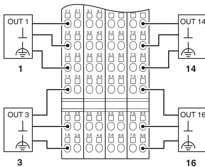
Disegno collegamento
