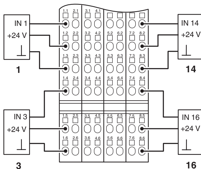
Disegno collegamento
