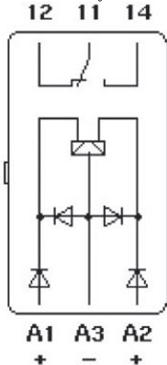
Schema di collegamento
