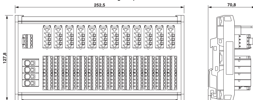
Disegno quotato
