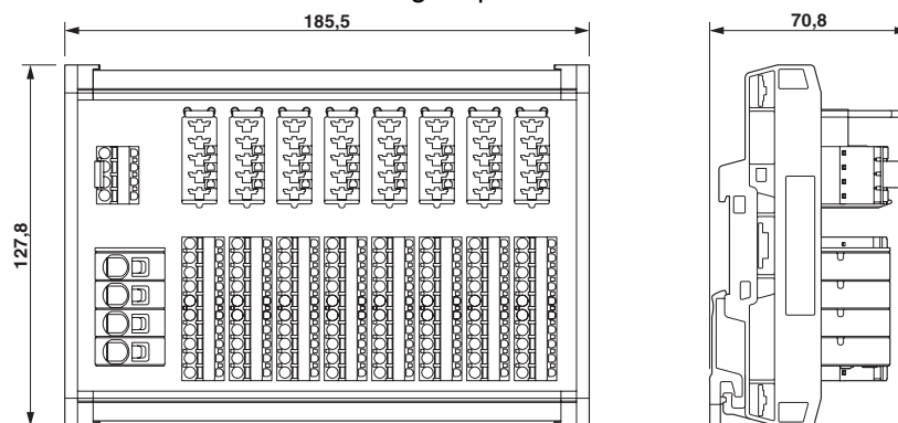
Disegno quotato
