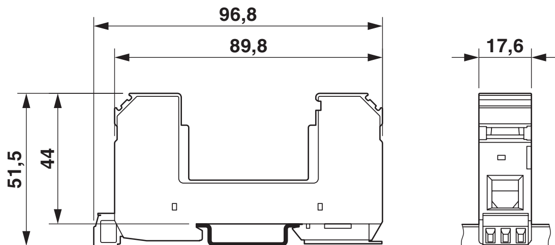
Disegno quotato
