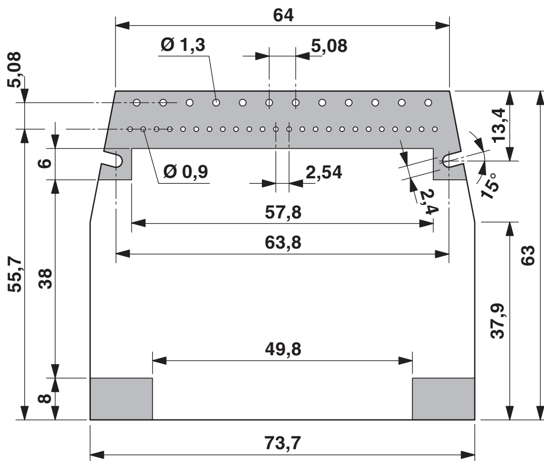
Disegno quotato
