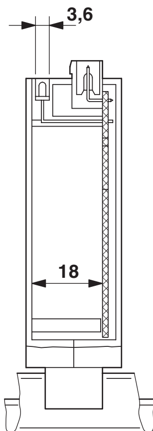
Disegno quotato
