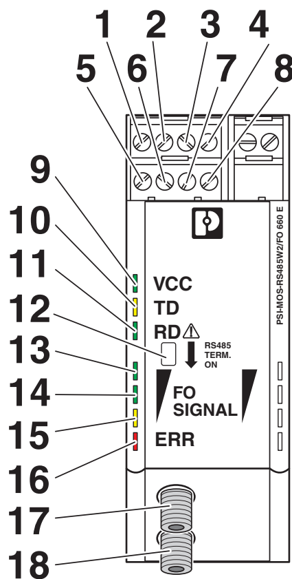
Disegno schema
