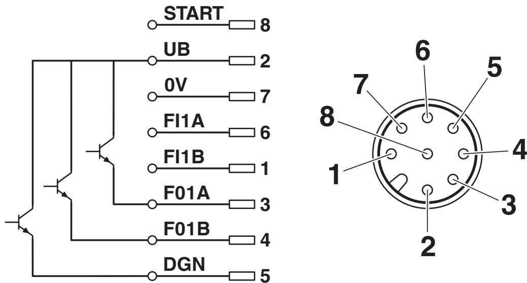
Disegno collegamento
