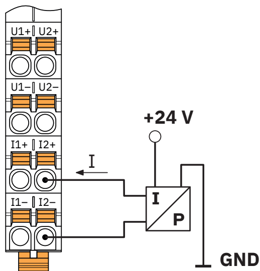
Disegno collegamento
