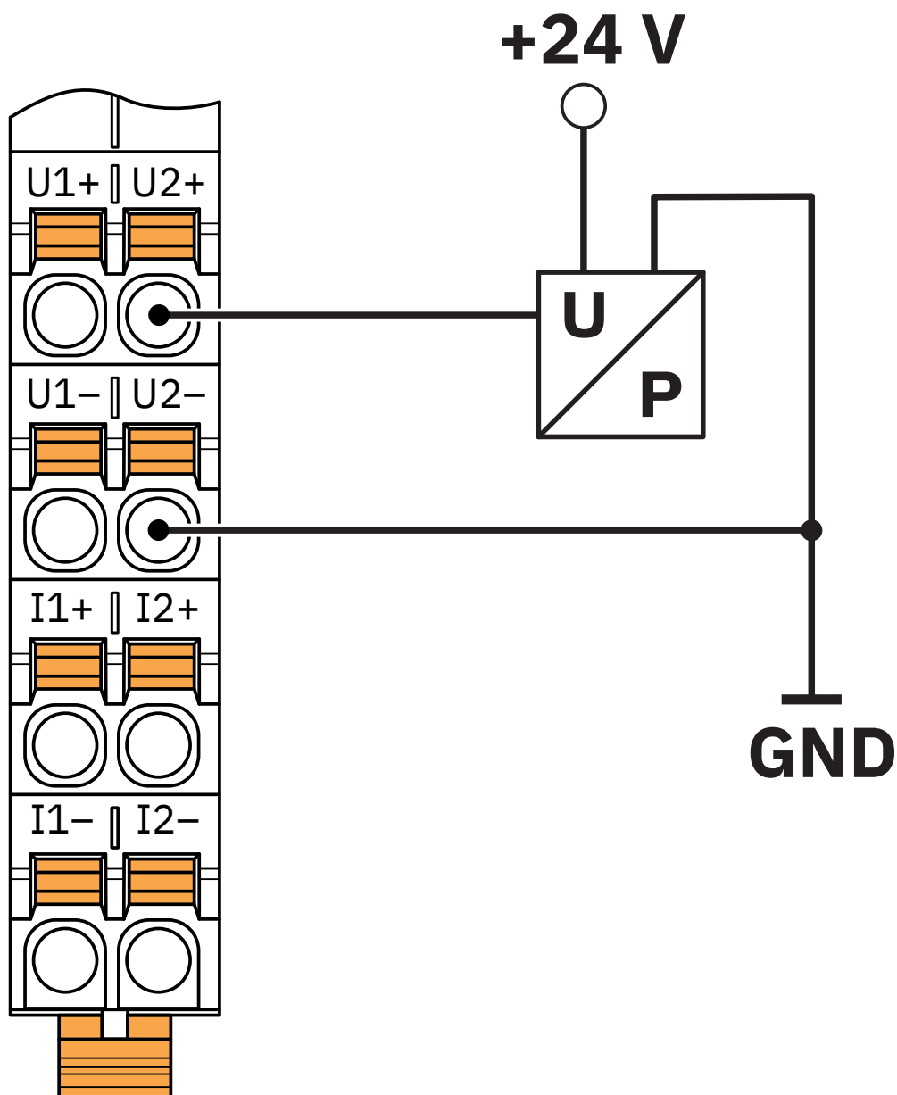
Disegno collegamento
