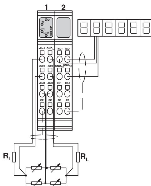
Disegno collegamento
