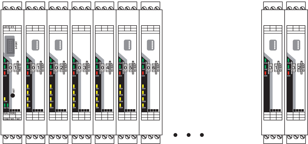
Stazione di collegamento Radioline con massimo 32 moduli di espansione I/O
