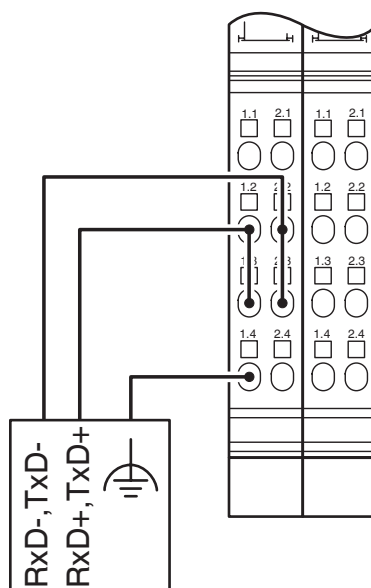
Disegno collegamento
