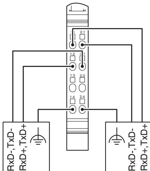
Disegno collegamento
