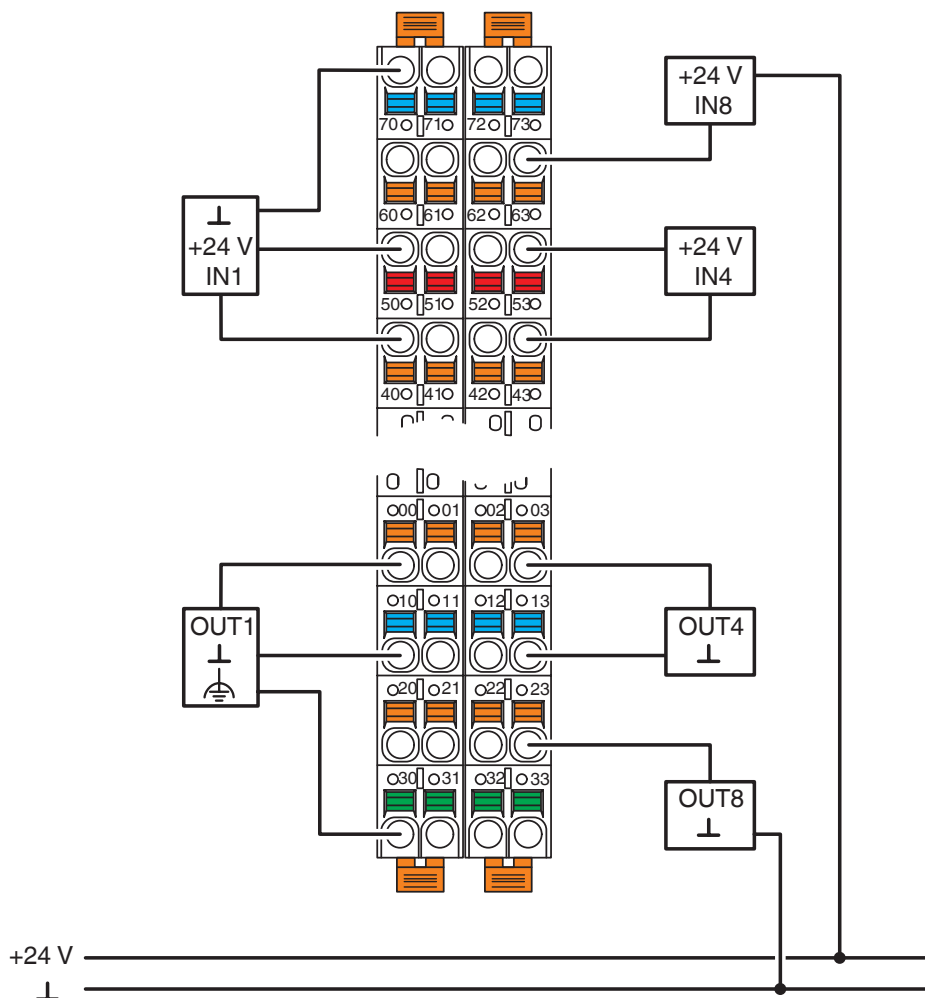
Disegno collegamento
