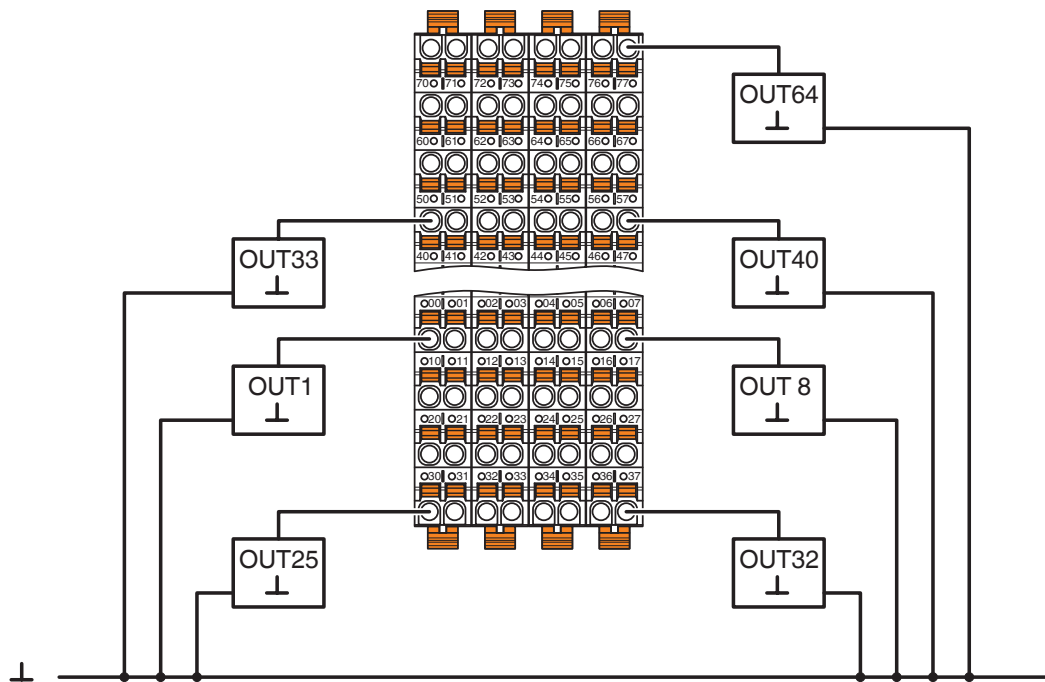
Disegno collegamento
